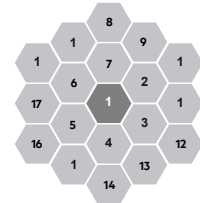
낮은 주파수 재사용 (w/ 20MHZ CHANNELS)
